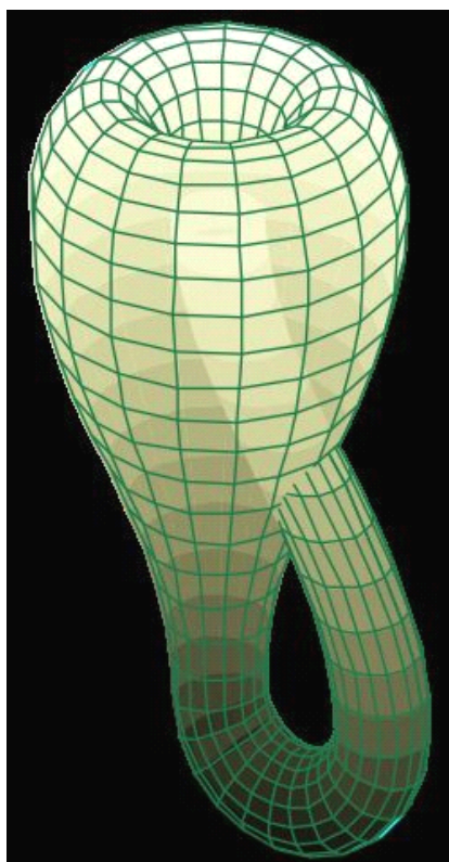
增图二：克莱因瓶
