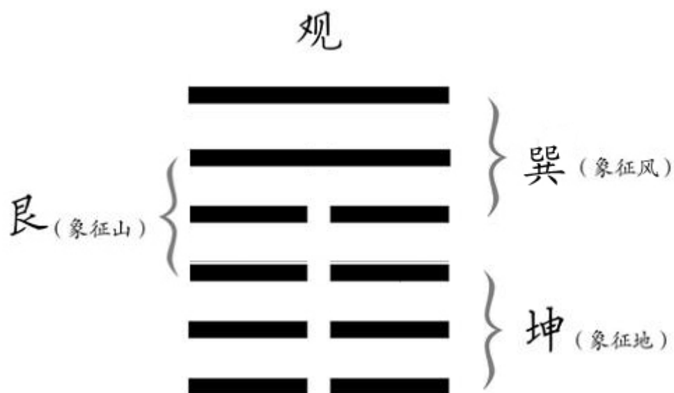
图16 – 观卦的互体
