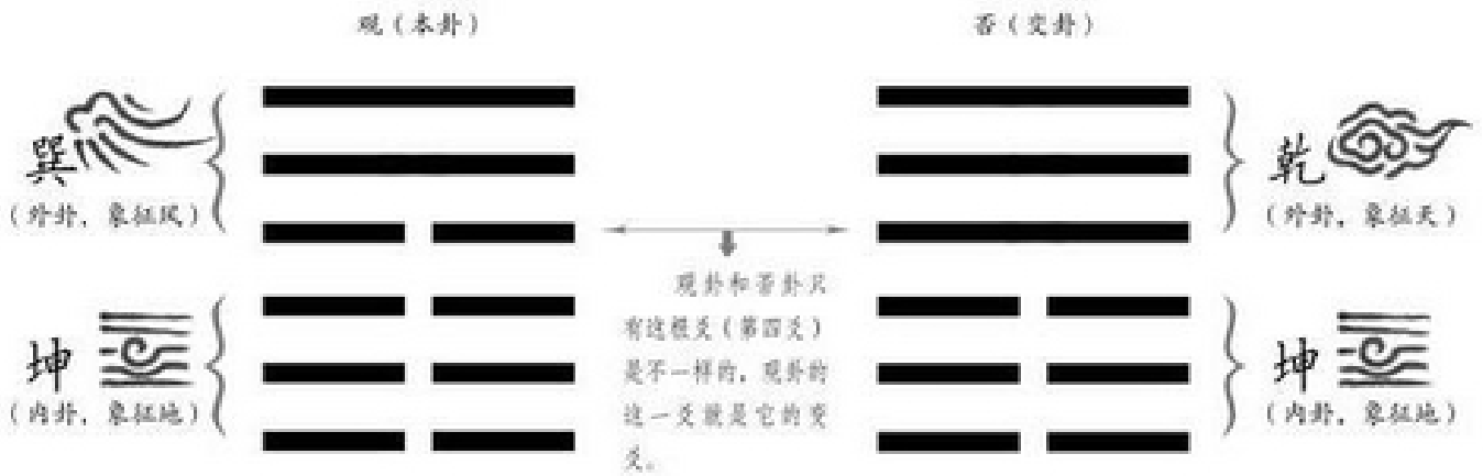
图15-观之否
