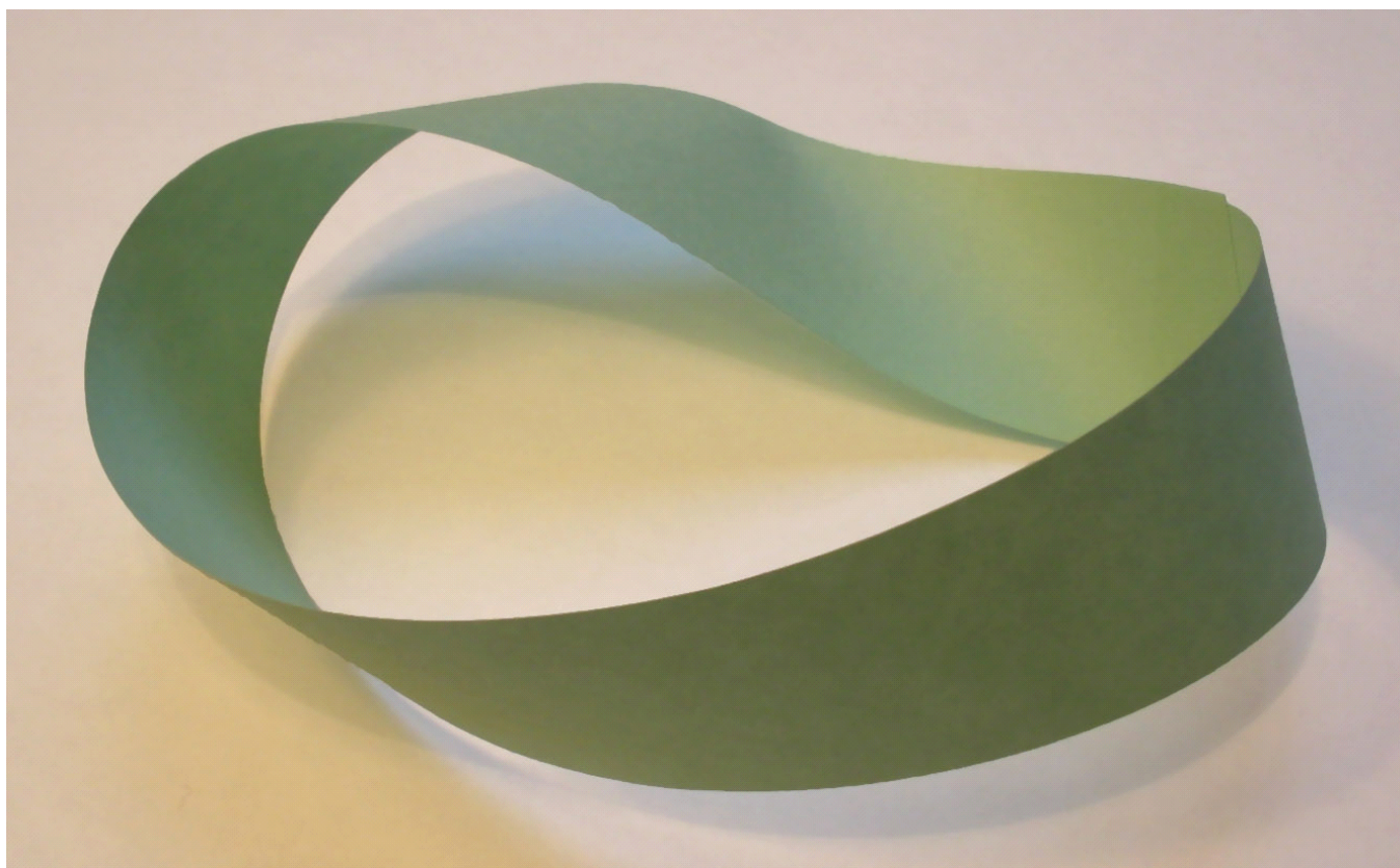
增图一：麦比乌斯带
