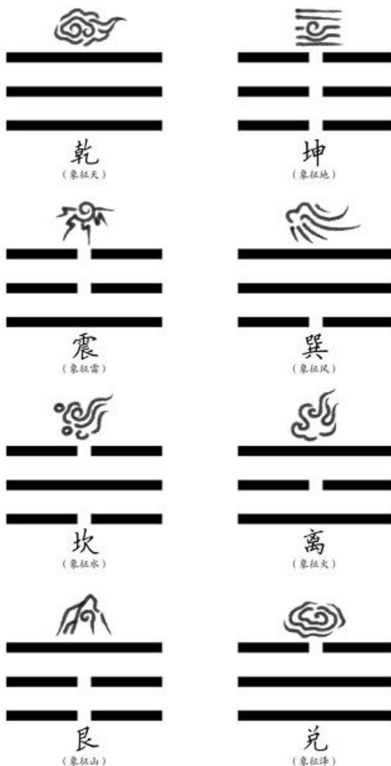
图8 - 八卦示意图
